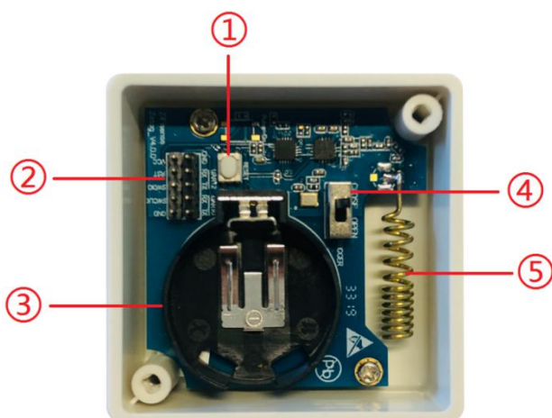
图 2：ZETag 广域云标签-ZETAG-C2 内部结构图
