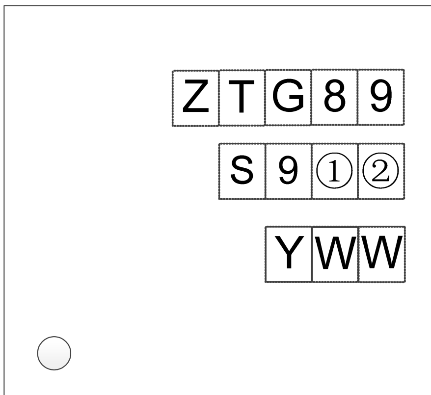
图 7-1. ZTG2189D 顶部丝印
