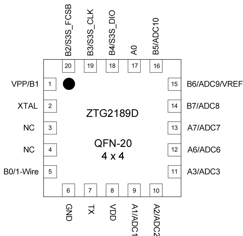
图 2-1. ZTG2189D QFN20 管脚排列
