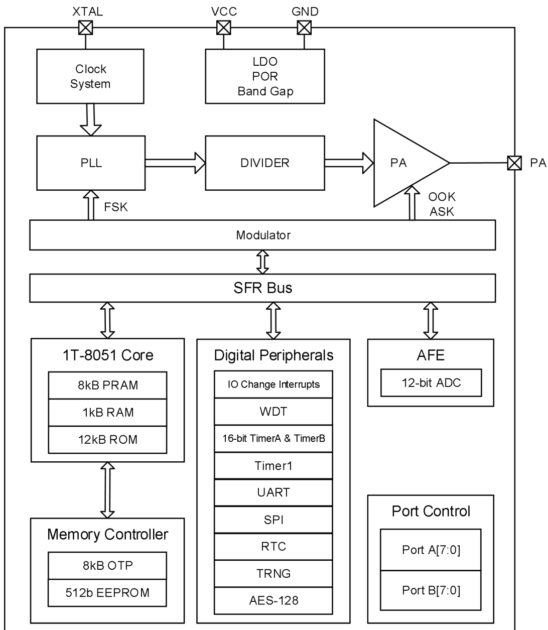
图 4-1. 系统框图
